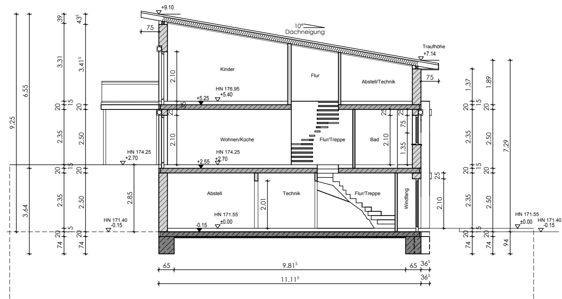
Schnitt A-A - Haus 1+2
